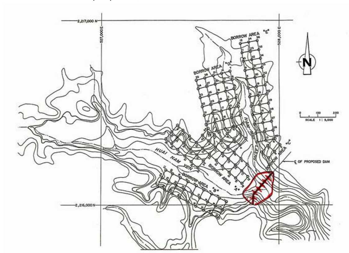
รูปที่ 5-1 ตัวอย่างแผนการเจาะสำรวจบ่อขุดดินในการก่อสร้างเขื่อน
